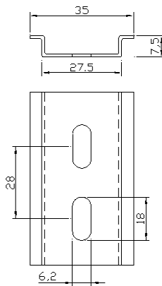
Aluminium Din Rail
