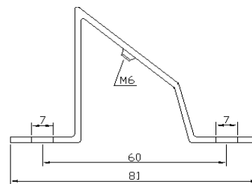
Din Rail Angle Bracket
