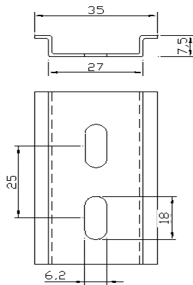
Steel Din Rail
